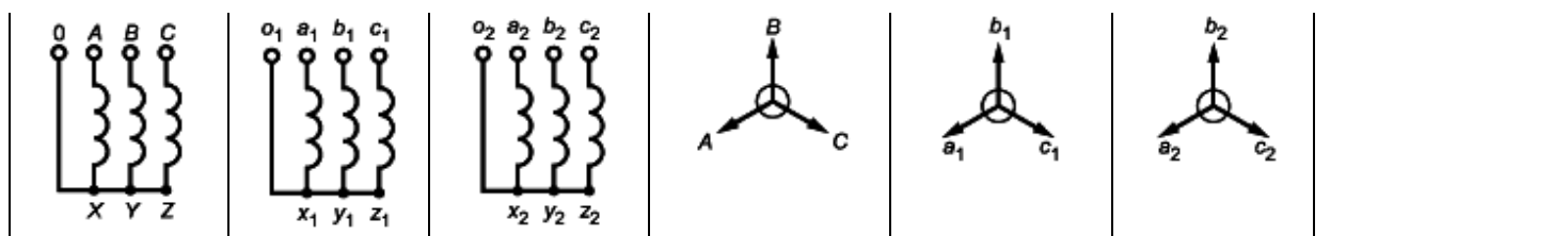
5.11 Условное обозначение трансформатора
